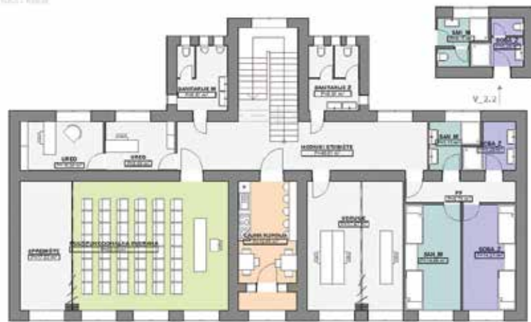
Idejni projekt rekonstrukcije Stare škole u Studeni (prvi kat)
